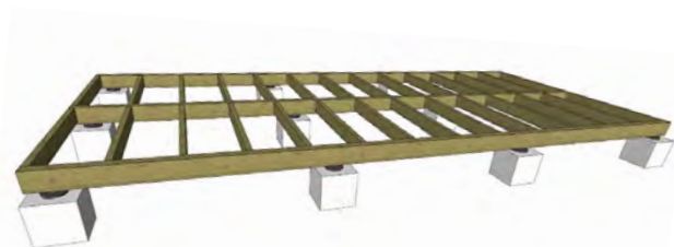
Support structure en bois
